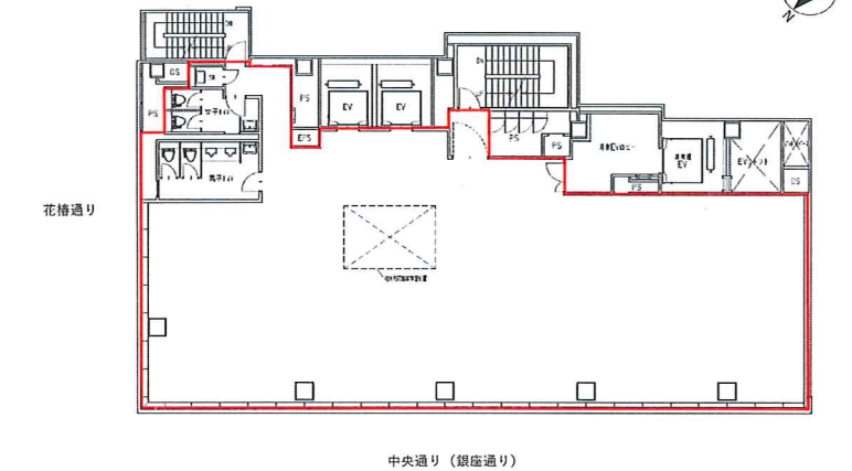
【3F平面図】
